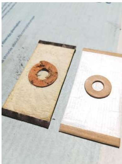
Porównanie mieszków od strony otworu wlotowego
